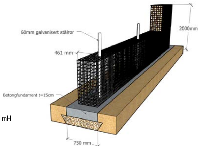
Frittstående mur over H=2m av 2mL x 0,5mB x 1,0mH
