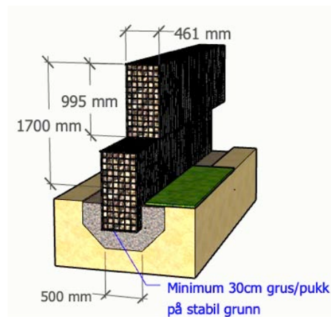
Frittstående mur H=1,7m av 2mL x 0,5mB x 1,0mH
